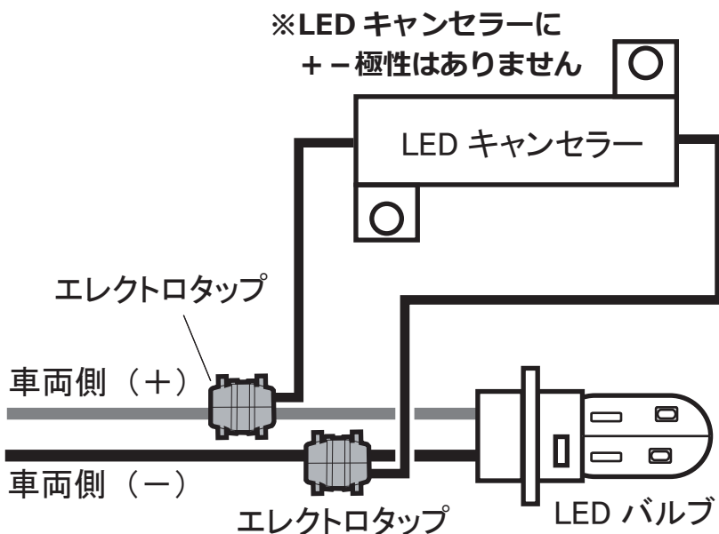
LED キャンセラー接続図（並列接続）
